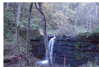
治山ダムの老朽化状況
