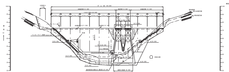
ダム背面図 S:1/1000
