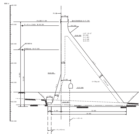
非越流部標準図 S:1/400
