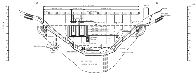
ダム正面図 S:1/1000
