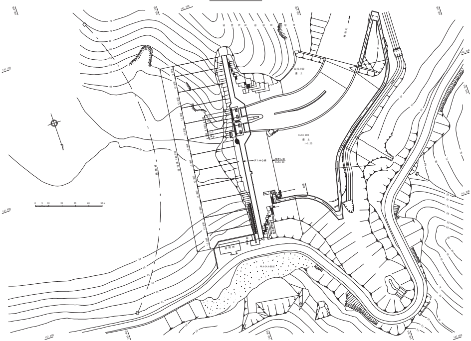
平面図 S:1/1000
