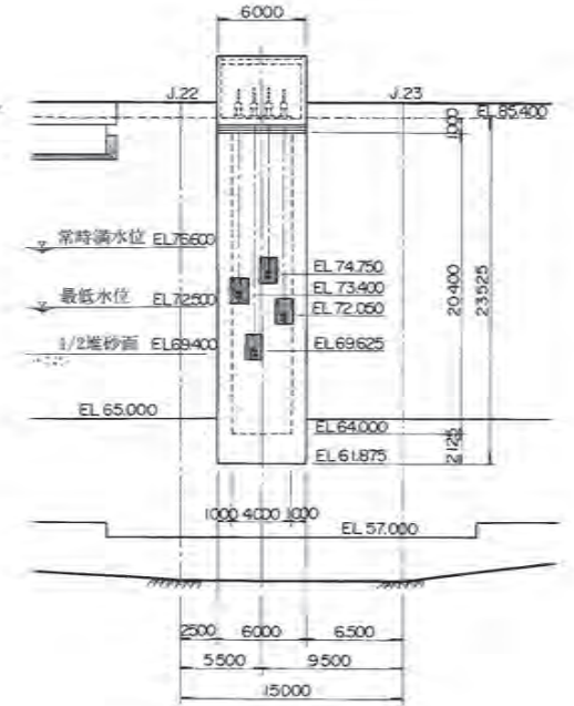
上流面図
