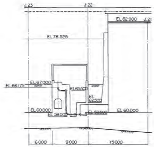
上流面図
