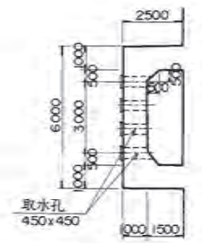
B-B断面
