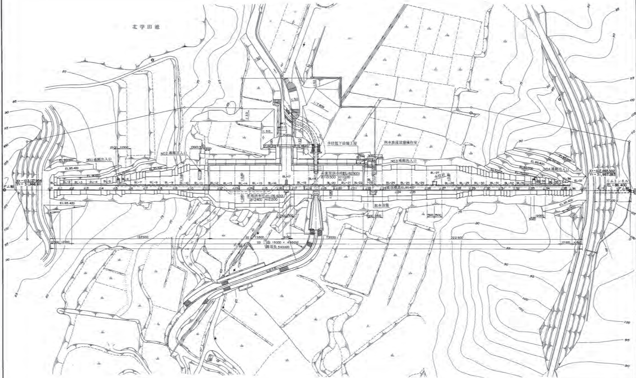
ダム本体 概要 ダム平面図
