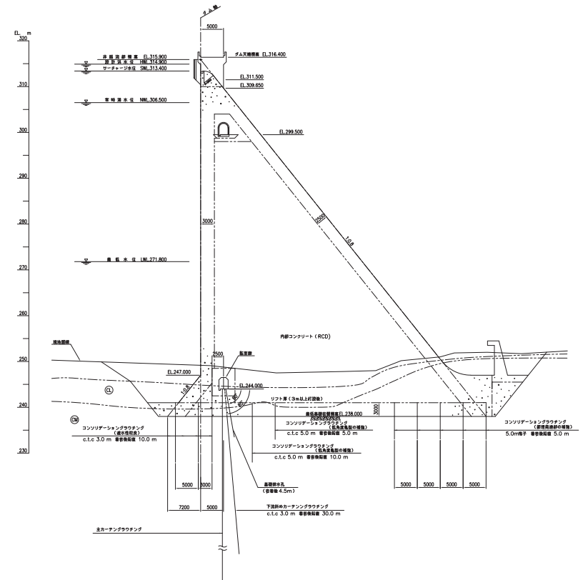
非越流部
