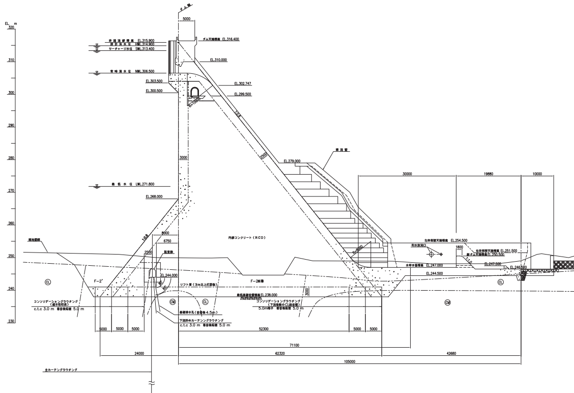
越流部 J10
