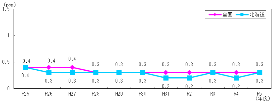
図 3-13 一酸化炭素濃度の年平均値の経年変化 [自動車排出ガス測定局]
