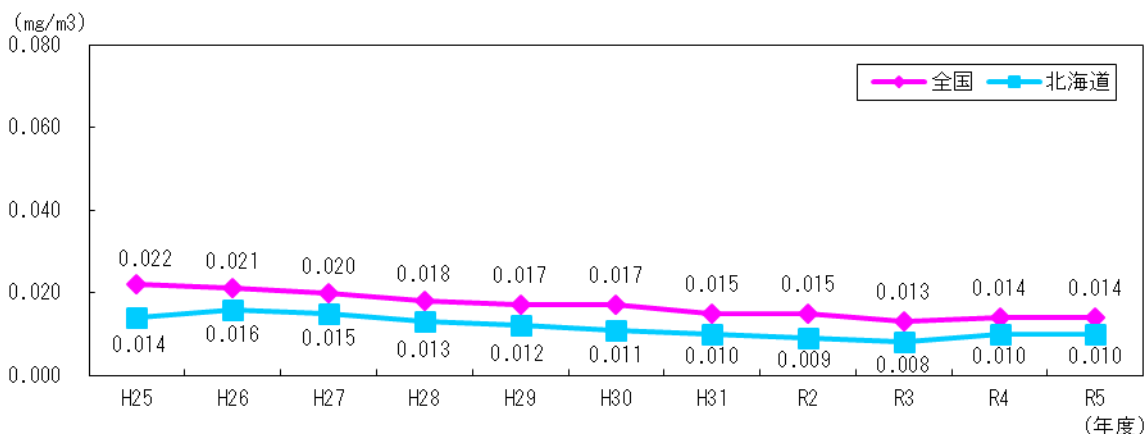
図 3-15 浮遊粒子状物質濃度の年平均値の経年変化 [自動車排出ガス測定局]
