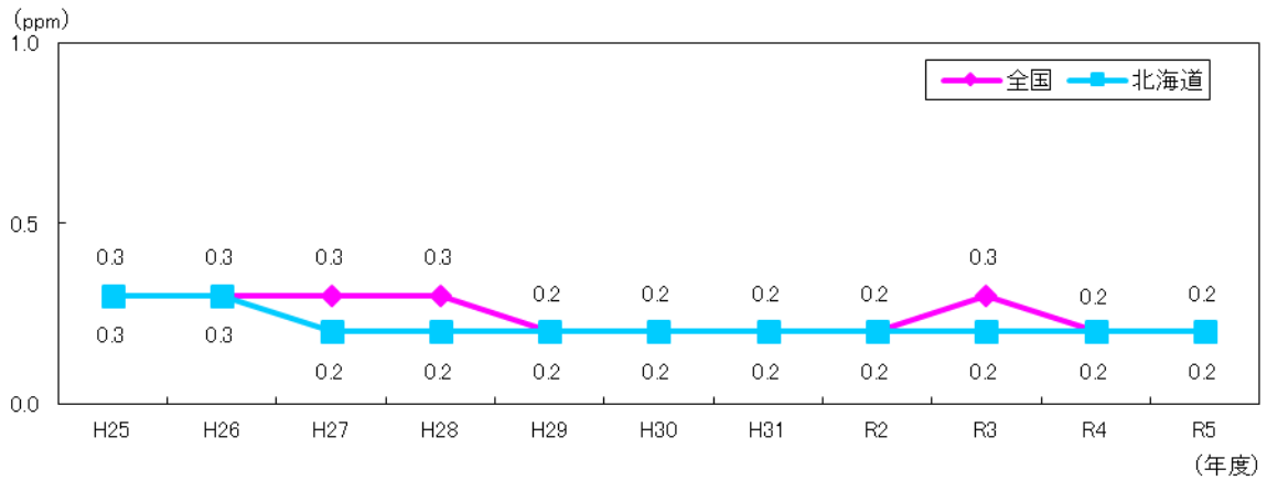
図 3-5 一酸化炭素濃度の年平均値の経年変化 [一般環境大気測定局]
