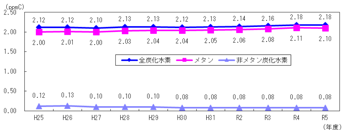
図 3-9 炭化水素濃度の年平均値の経年変化 [一般環境大気測定局]
