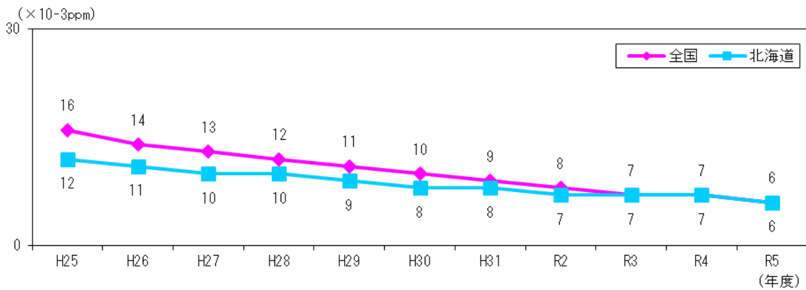
図 3-11 一酸化窒素濃度の年平均値の経年変化 [自動車排出ガス測定局]
