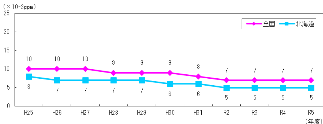
図 3-4 二酸化窒素濃度の年平均値の経年変化 [一般環境大気測定局]
