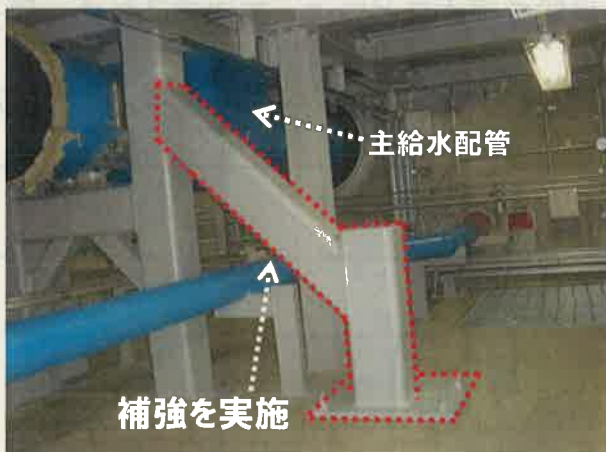
《耐震補強工事の例》
