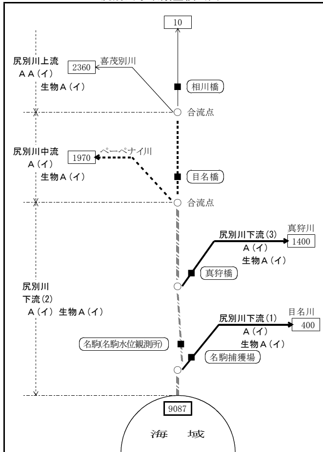
尻別川水域類型模式図
