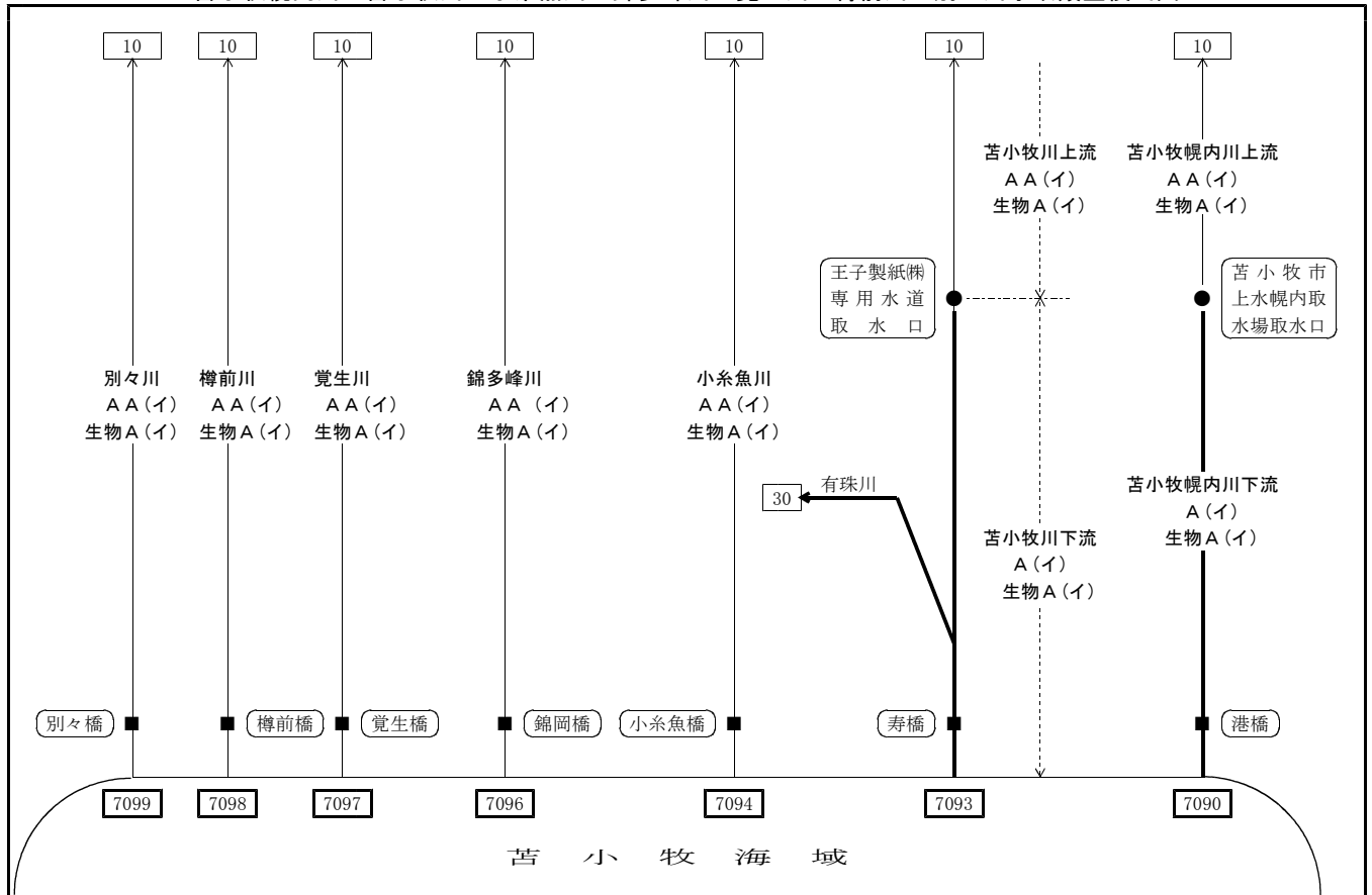
苦小牧幌内川・苦小牧川・小糸魚川・錦多峰川・覚生川・樽前川・別々川水域類型模式図
