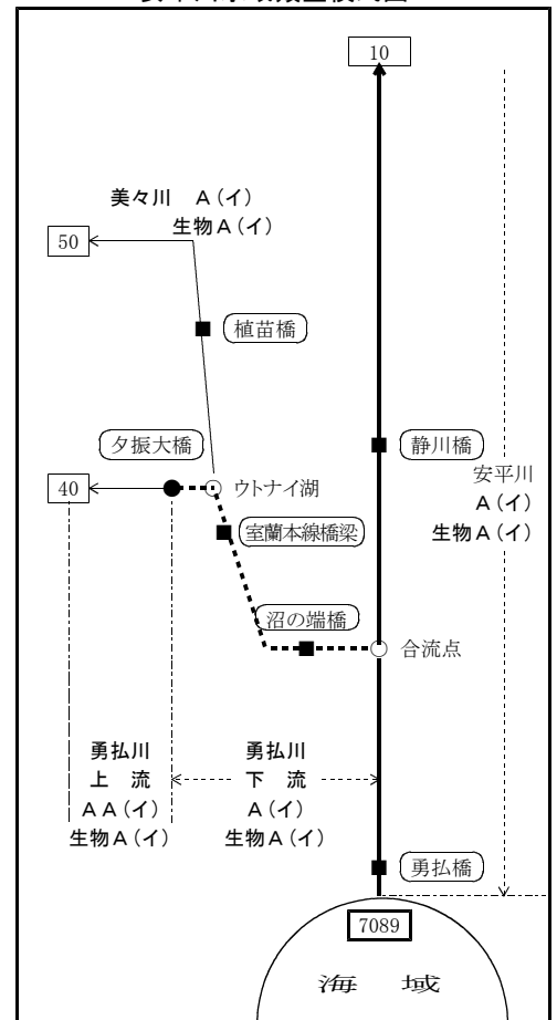
安平川水域類型模式図
