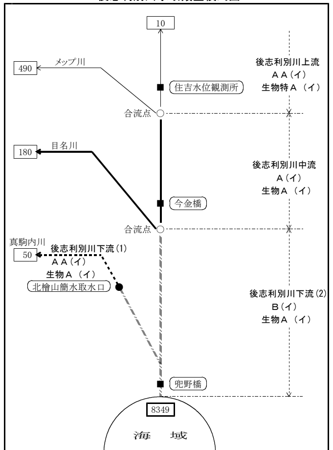
後志利別川水域類型模式図
