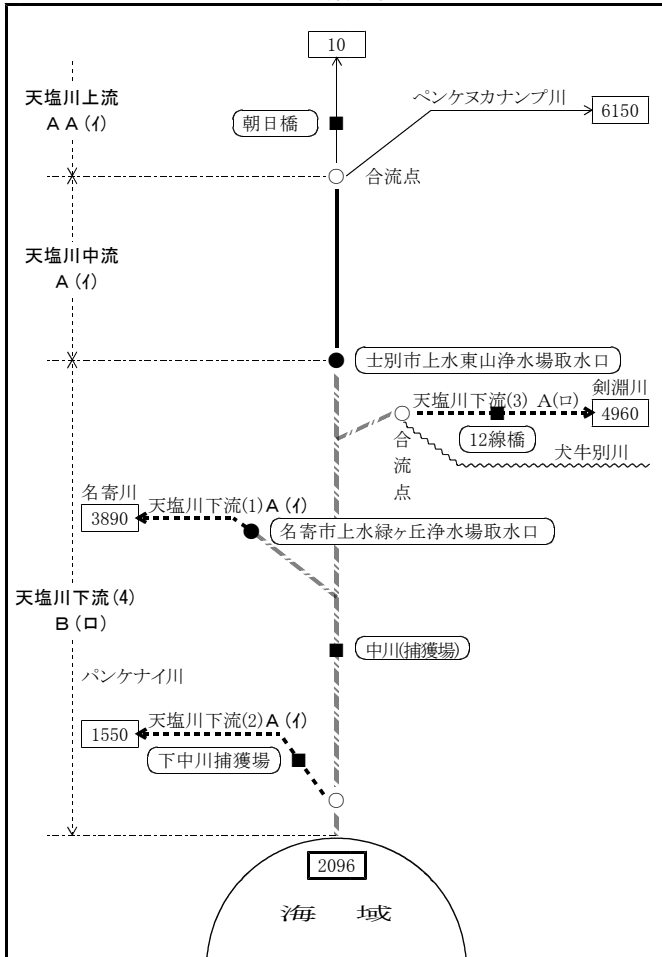
天塩川水域類型模式図
