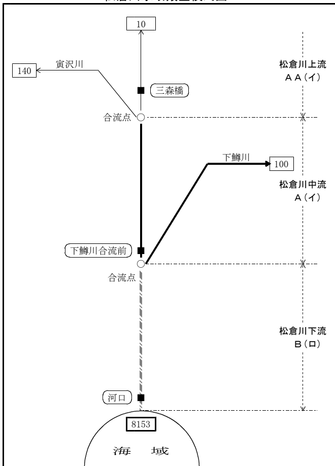
松倉川水域類型模式図
