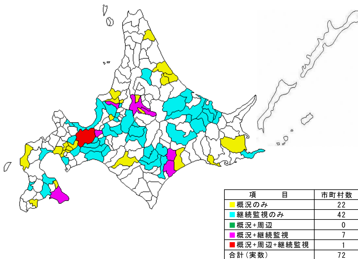
図1 令和元年度地下水の水質調査地点（市町村別、実施調査別）
