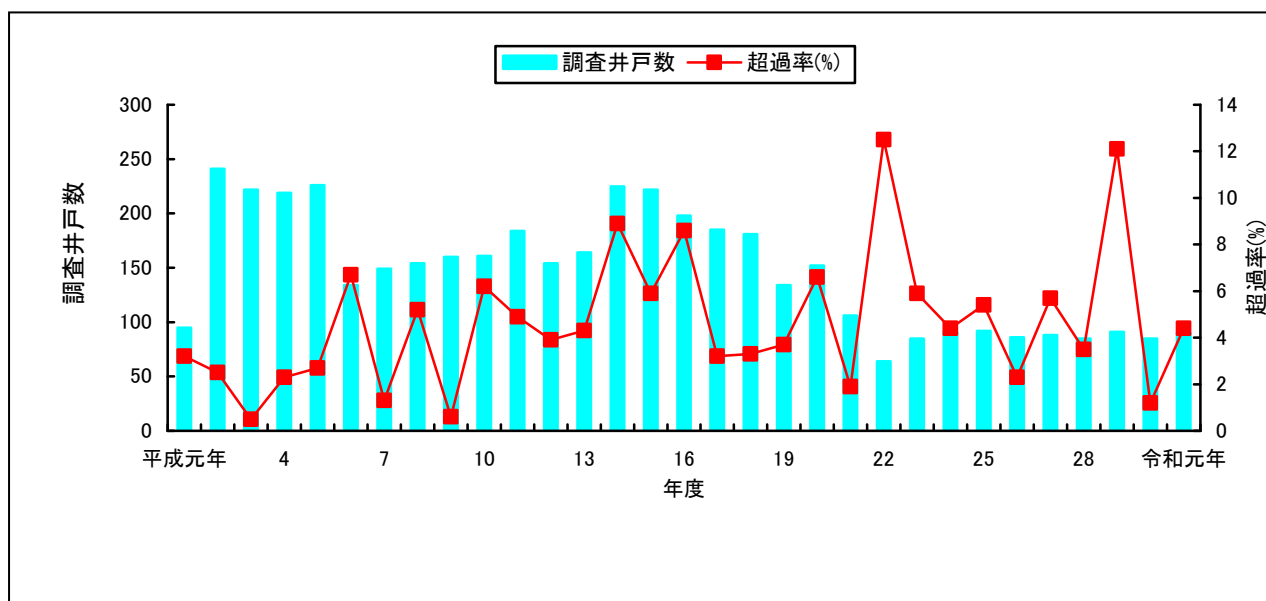
図2 年度別概況調査井戸数と超過率の推移
